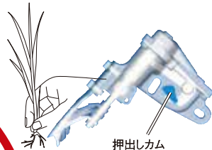
押し出しカム
